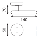
art. MA 2.5570 guarnitura rosetta e bocchetta bombata ø 50 mm ad avvitare
