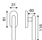
art. FI 2.5460 dk movimento in fibra
