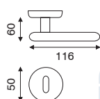
art. MA 2.5470 guarnitura rosetta e bocchetta bombata ø 50 mm ad avvitare
