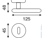
art. MA 2.1661 BIC guarnitura rosetta e bocchetta ø 45 mm a pressione
